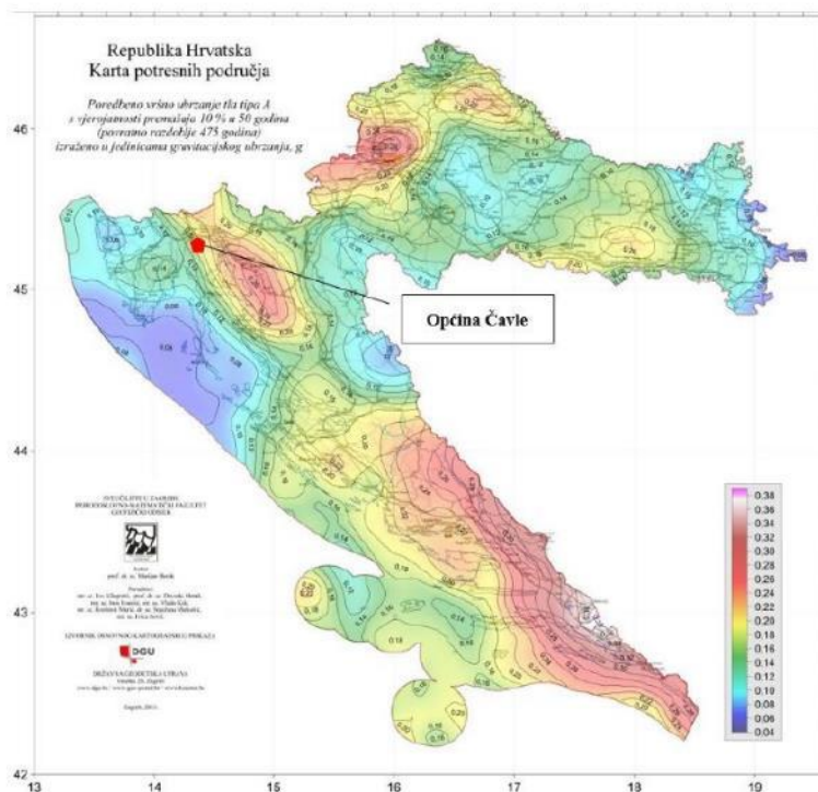
Slika 1. Vršna ubrzanja tla uzrokovana potresima za područje Općine Čavle za povratni period za 475 godina
