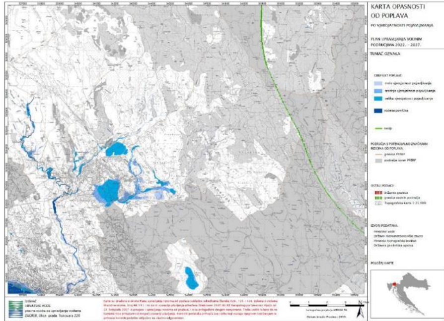
Slika 2. Pregledna karta opasnosti od poplava po vjerojatnosti pojavljivanja za područje Općine Čavle
